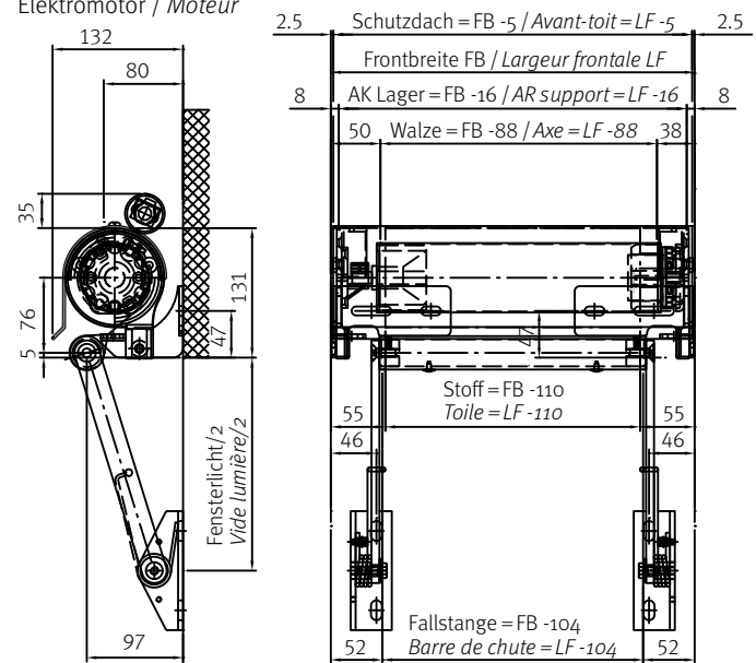
Befestigung Arme Fassade / Walzenkonsole ins Zwischengewände Fixation des bras en façade / Supports en embrasure Elektromotor / Moteur
