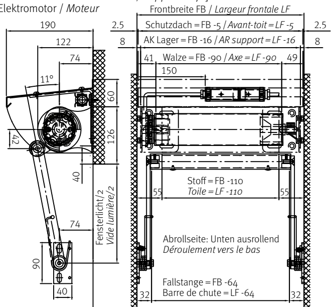
Führung an Fassade / Walzenkonsole an Fassade / Arme mit Ausstellfeder Fixation des bras en façade / Supports en façade / Bras avec ressorts Elektromotor / Moteur
