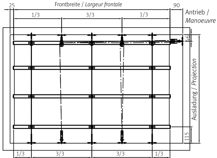
Grundriss / Plan
