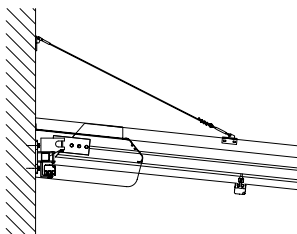
Wandabspannung für Anlagen mit mehr als 9 m Ausladung
