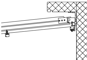
Montage unten an die Decke Montage sous dalle
