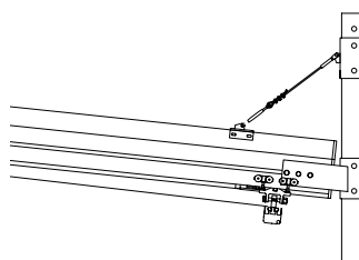
Stützenabspannung für Anlagen mit mehr als 9 m Ausladung
