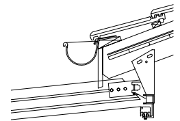
Dachsparrenmontage Montage sur chevron
