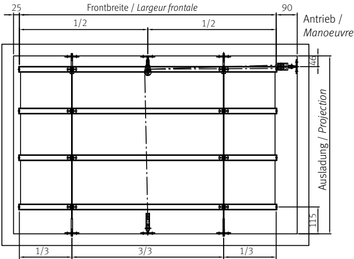
Grundriss / Plan
