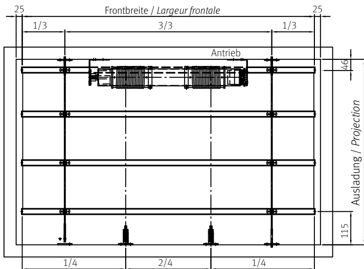
Grundriss / Plan
