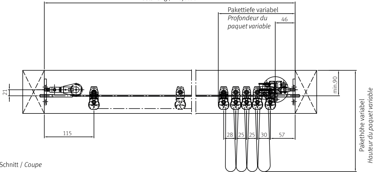
Ausladung / Projection
