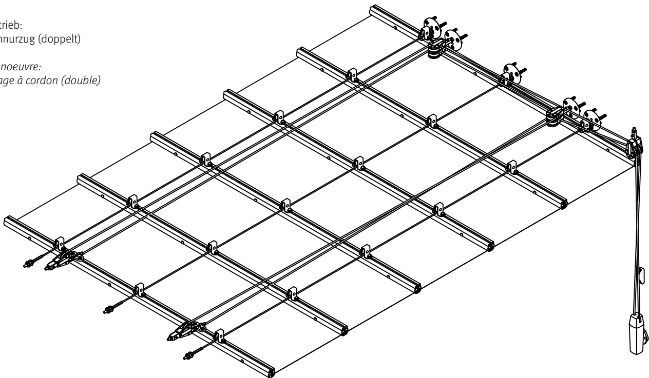
Ausladung / Projection
