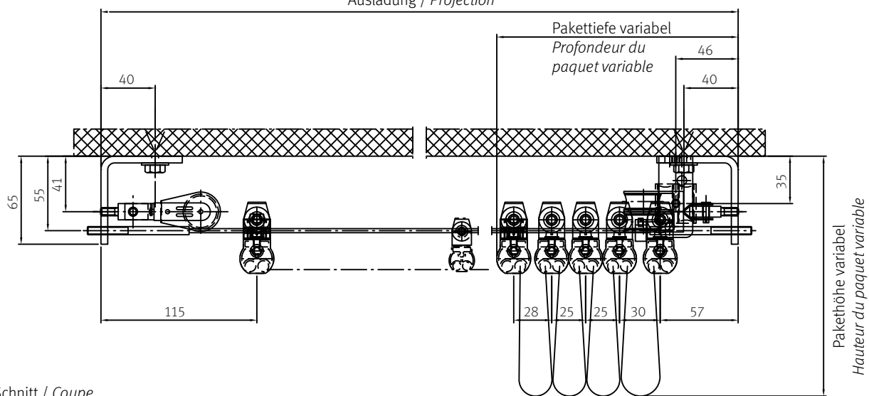
Schnitt / Coupe
