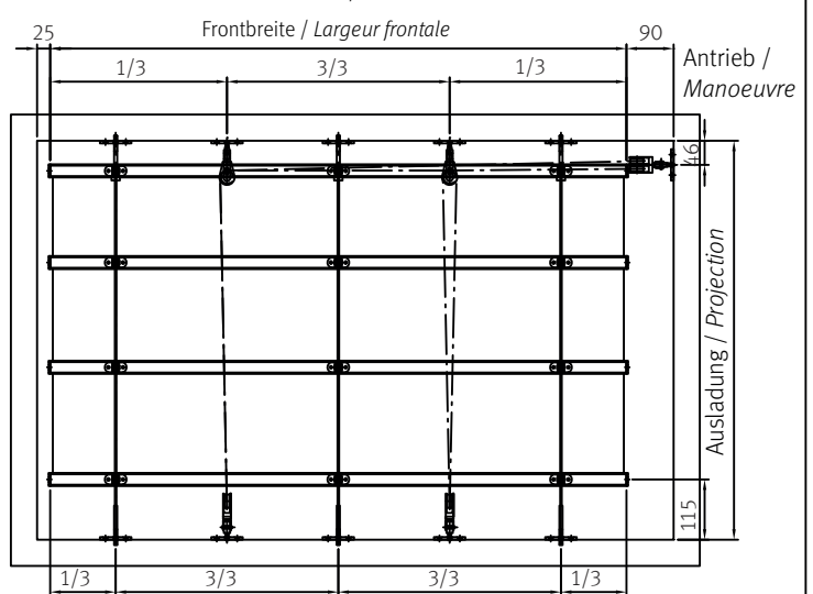
Grundriss / Plan
