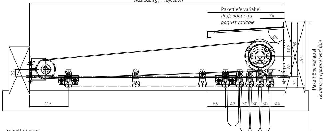
Schnitt / Coupe
