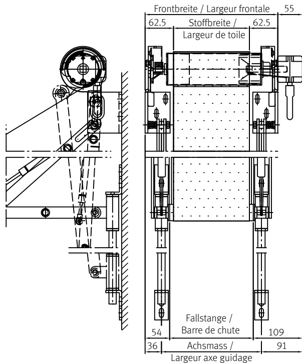
Führungslager Fassade unten Support guidage façade en bas
