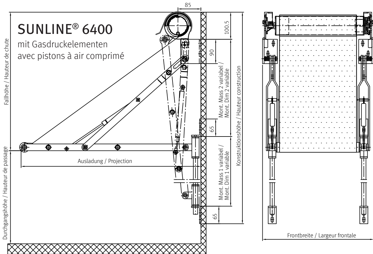
Montage an die Fassade / Montage en façade Elektromotor / Moteur
