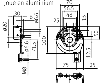
Gusskopf Joue en aluminium
