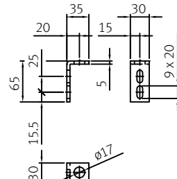
Führungslager Fassade unten Support guidage façade en bas
