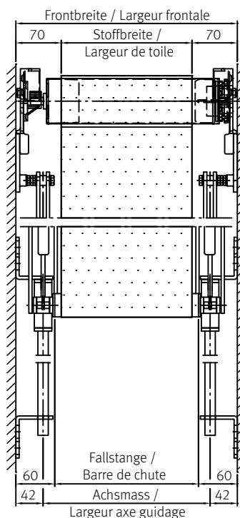
Führungslager Zwischengewände unten Support de guidage en embrasure en bas
