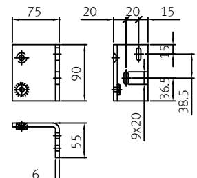
Montagewinkel Fassade zu Gusskopf Support montage façade
