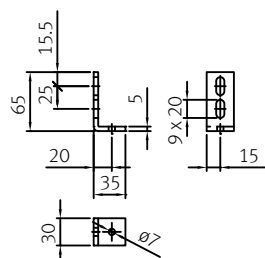
Führungslager Fassade oben Support guidage façade en haut
